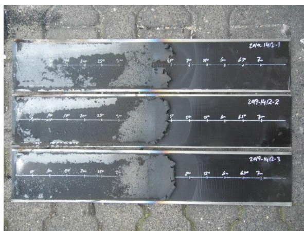
Aussehen der Proben nach dem Spread of Flame Versuch Appearance of the specimen after the spread of flame test
